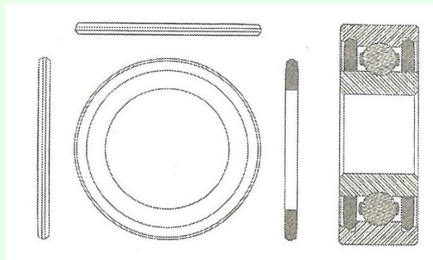
本件登録意匠
