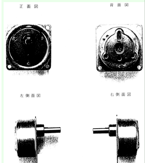
被告意匠中の 減速機部分
