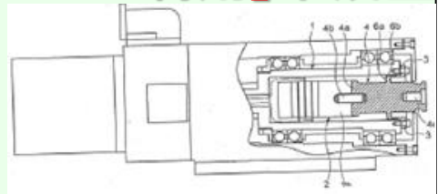
被告製品 （スピンドル）
